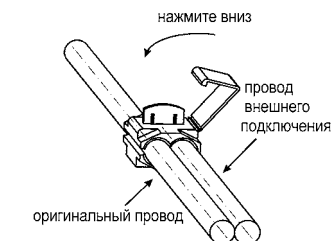
рис.5 Соединение проводов через зажим
